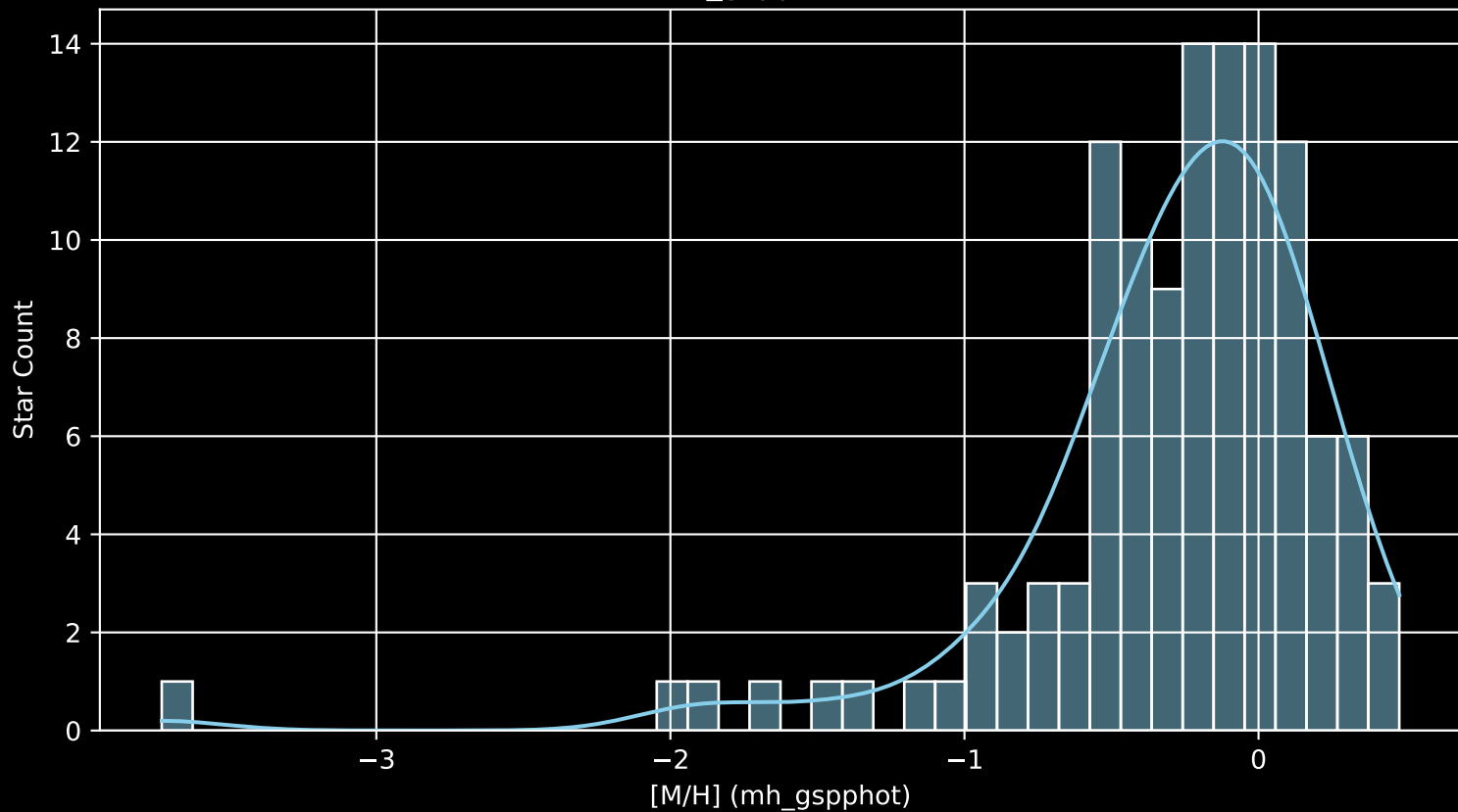
APOGEE DR17 Field: [281-35-O [M/H] (mh_gspphot) (n= 119)
