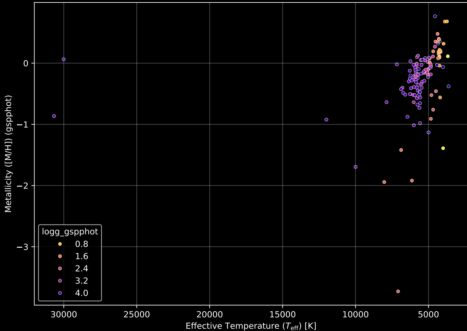
APOGEE DR17 Field: [281-35-O] Stellar Population Parameters (n= 122)
