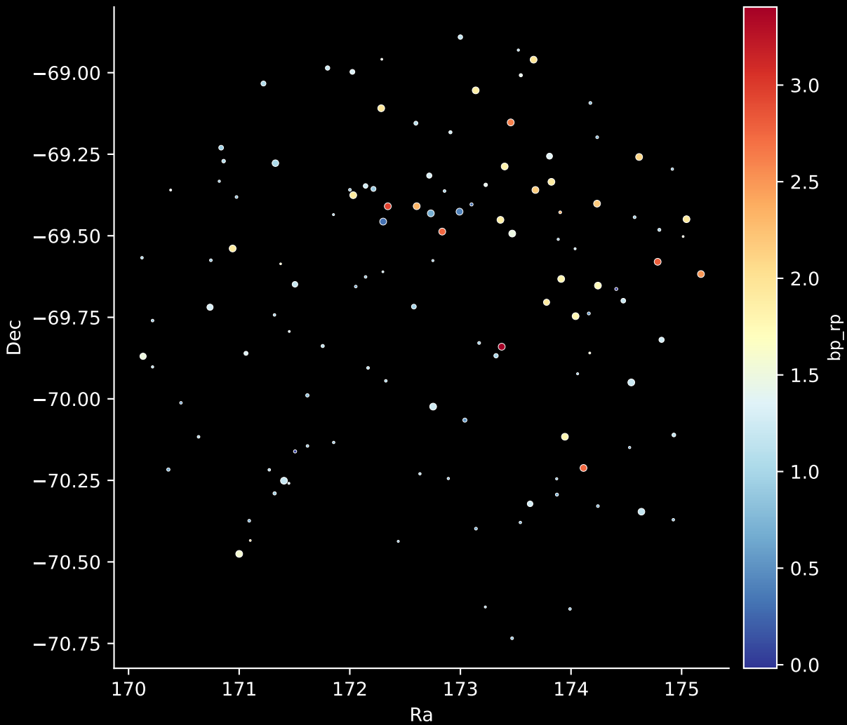
APOGEE DR17 Field: [281-35-O] Stars: 122
